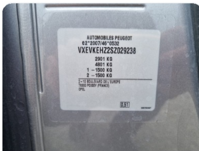
Tabliczka znamionowa
